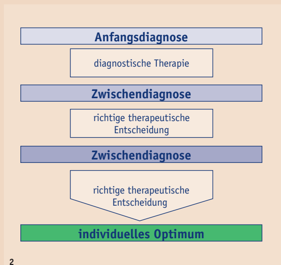
Abb. 2: Diagnostischer Pfad.
